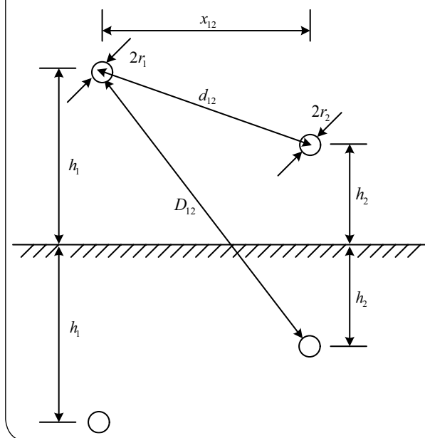
Рис.1. Провода и их зеркальные отражения (электрическое поле)
