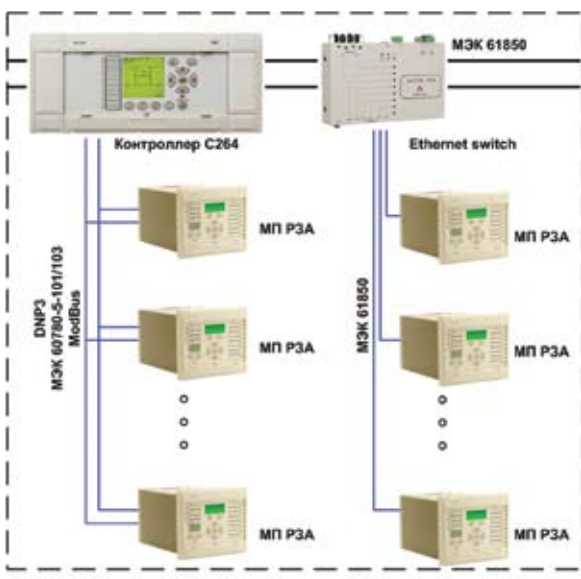
Архитектура системы PACIS с подключением микропроцессорных устройств РЗА через МЭК61850
