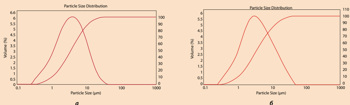
Рис. 1. Кривые распределения по размерам гидроокиси магния производства Италии (а) и отечественной (б)
