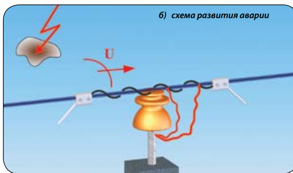
Рис. 4 Пережог провода на ВЛЗ, оборудованной дугозащитными рогами
